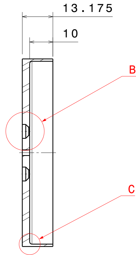
CORTE A-A
